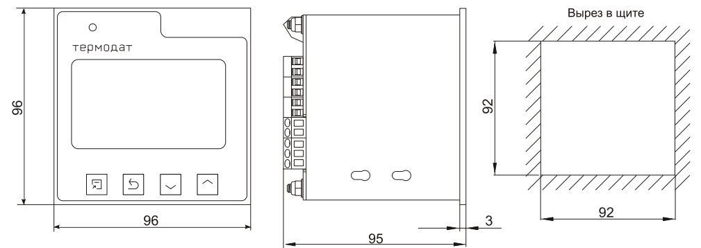
Основной блок
