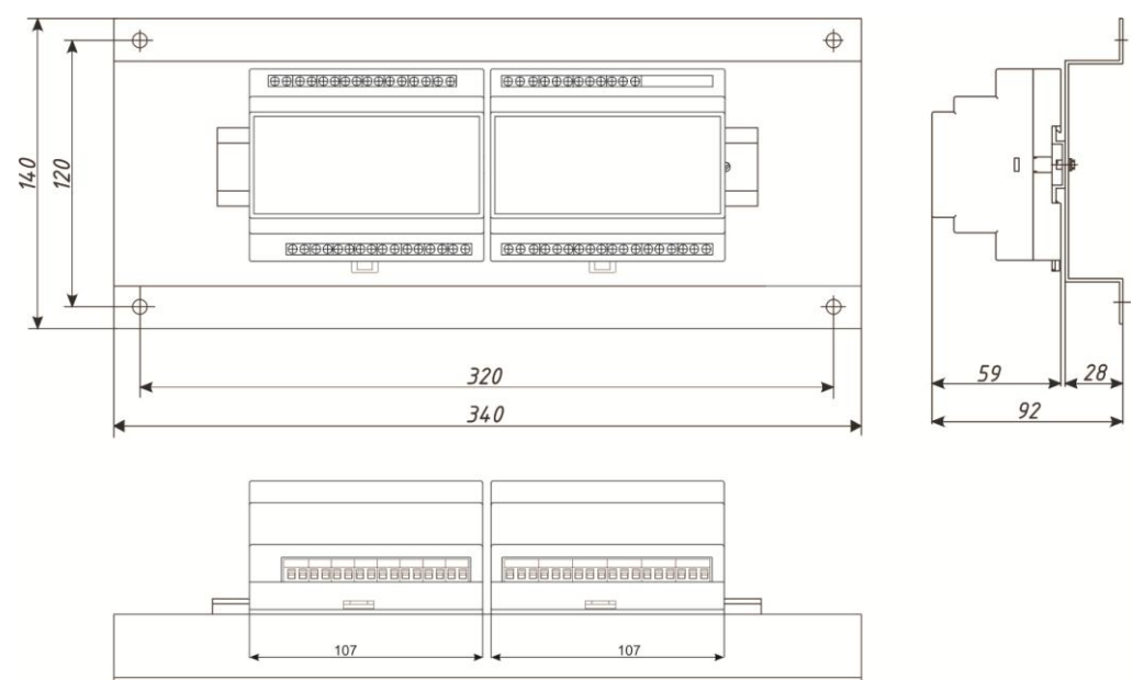
Периферийный блок
